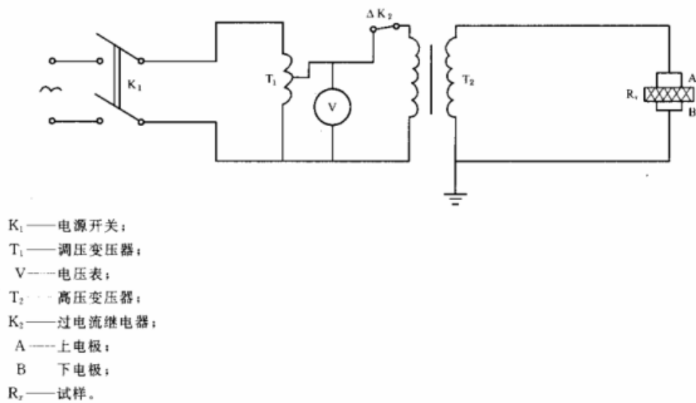
图 1 击穿电压测试原理图
